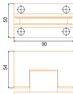
Bản lề kính 90 - Đôn 11083 (Glass Hinge)
