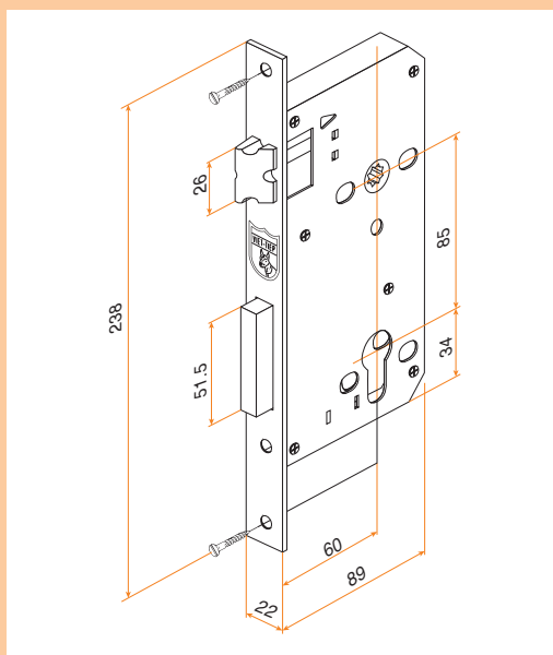
Hộp khóa 04292 Lock case 04292
