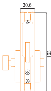
Khóa sàn 11046 (Floor lock)
